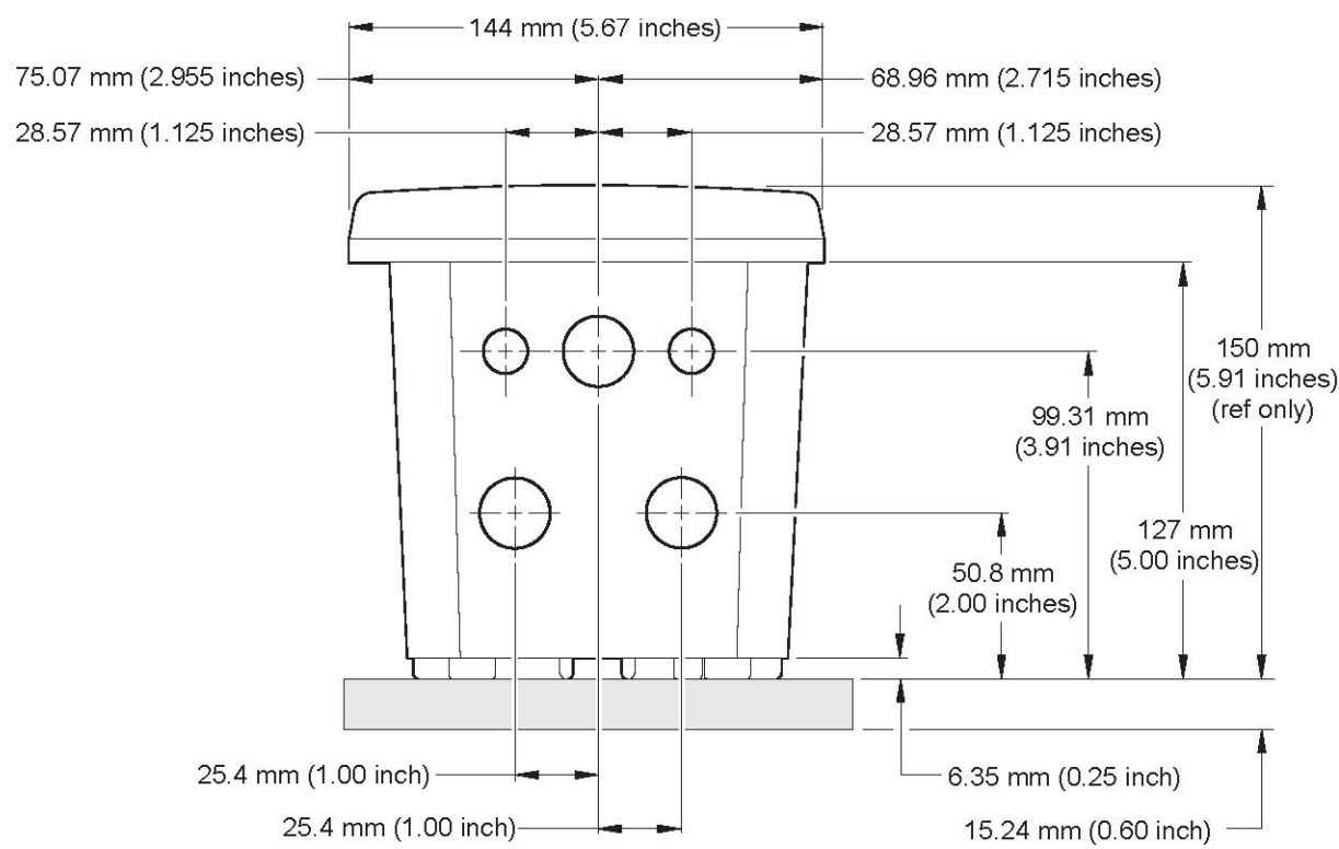
图6 导管孔尺寸
