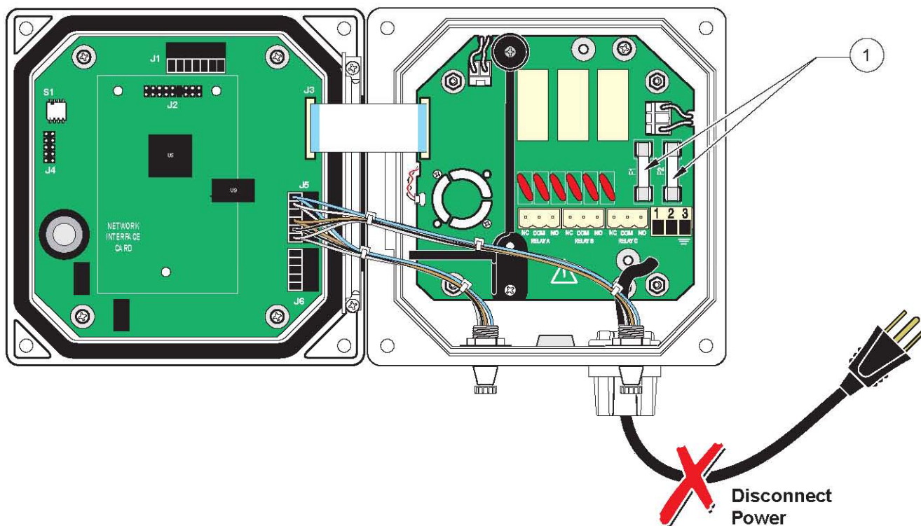
图37更换保险丝
