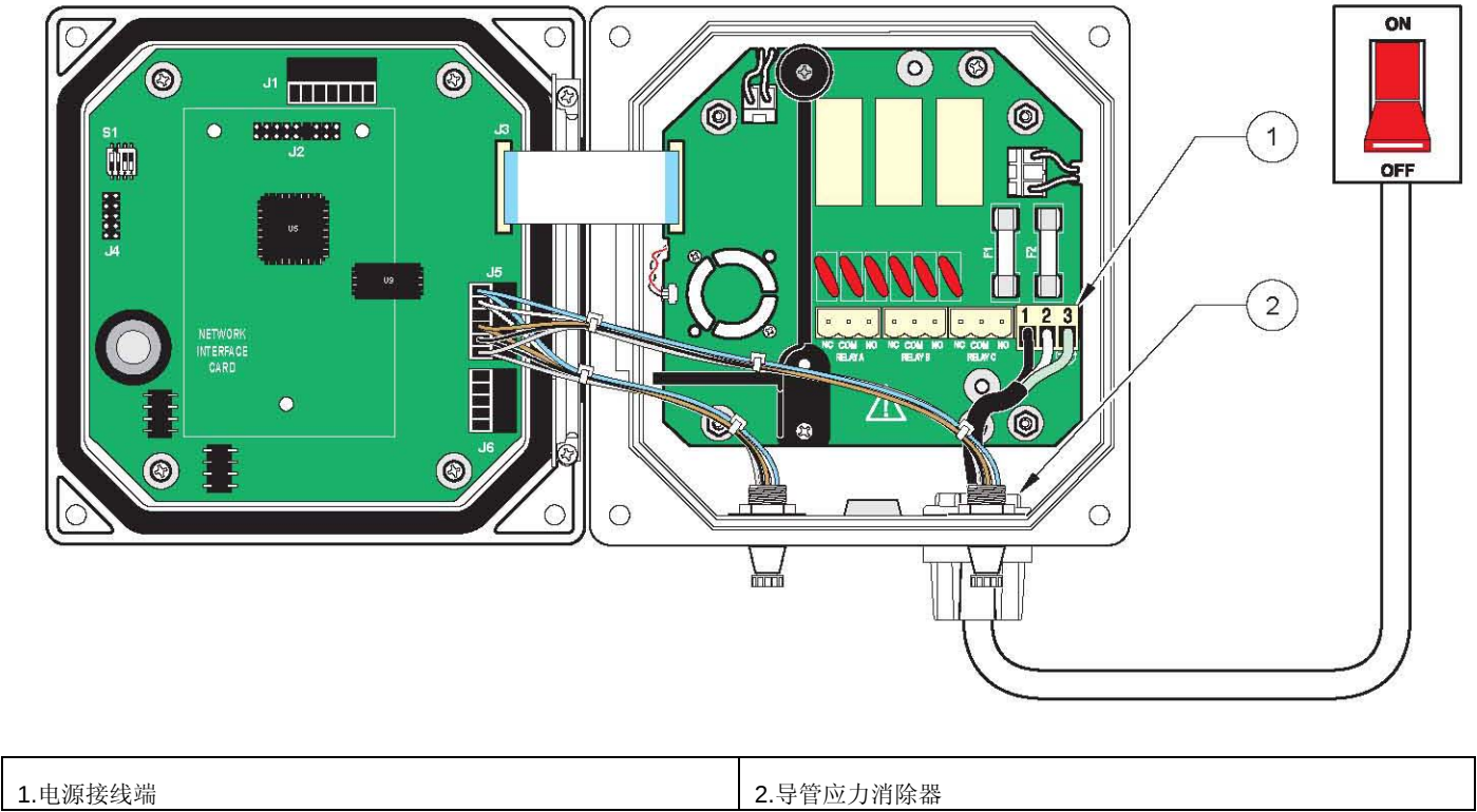
图17 硬导线连接电源局部断路开关
