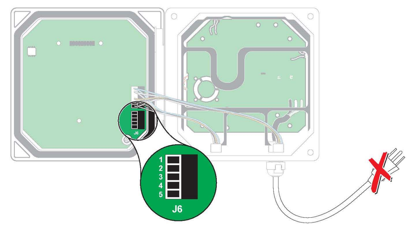
图19 模拟输出端口连接
