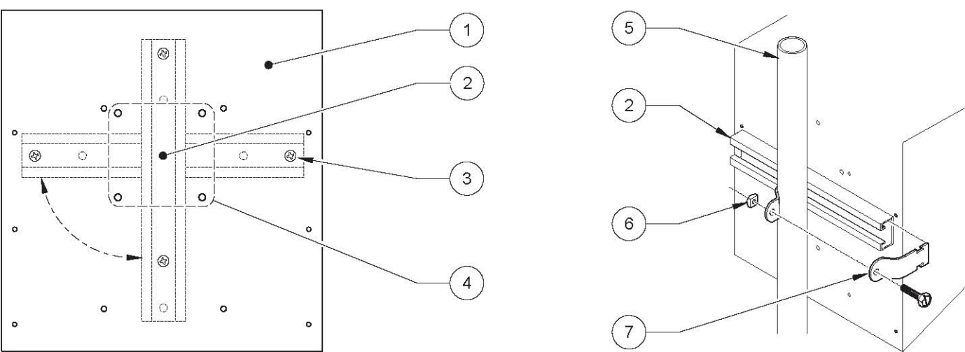
图8 遮阳罩内的控制器安装
