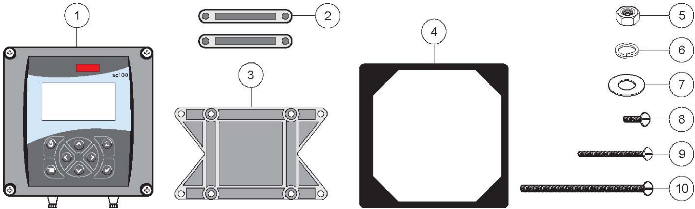
图2 控制器部件
