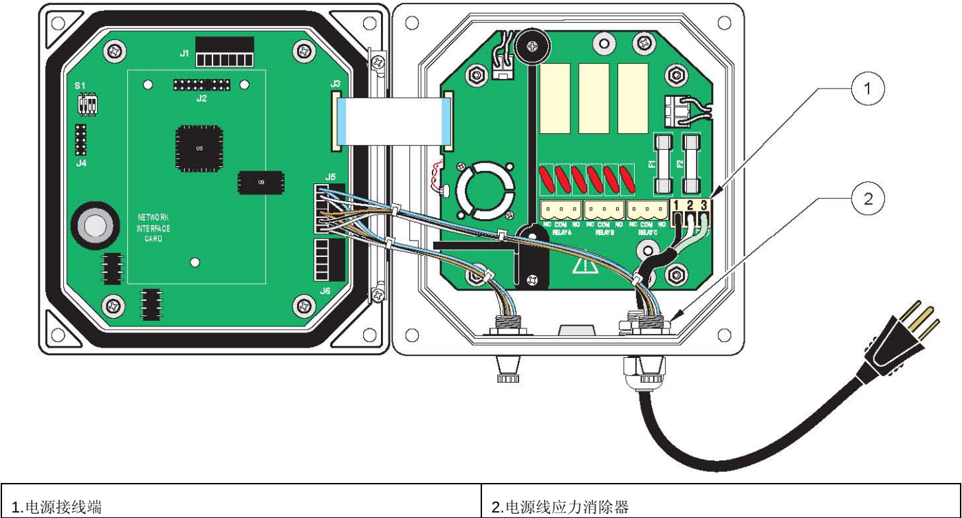
图16 电源线局部断路开关
