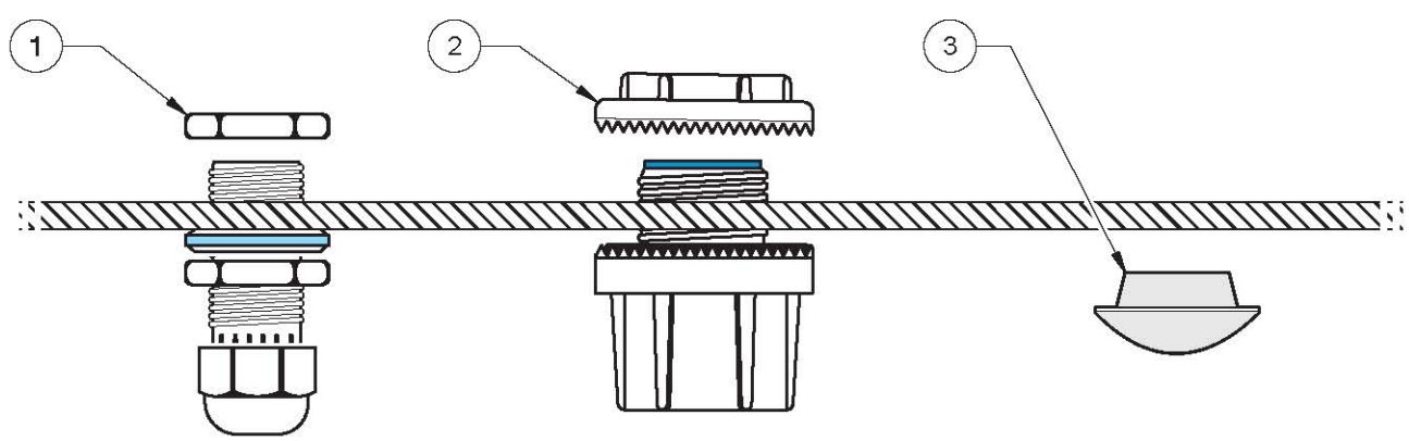
图13 可选应力消除器和导管塞
