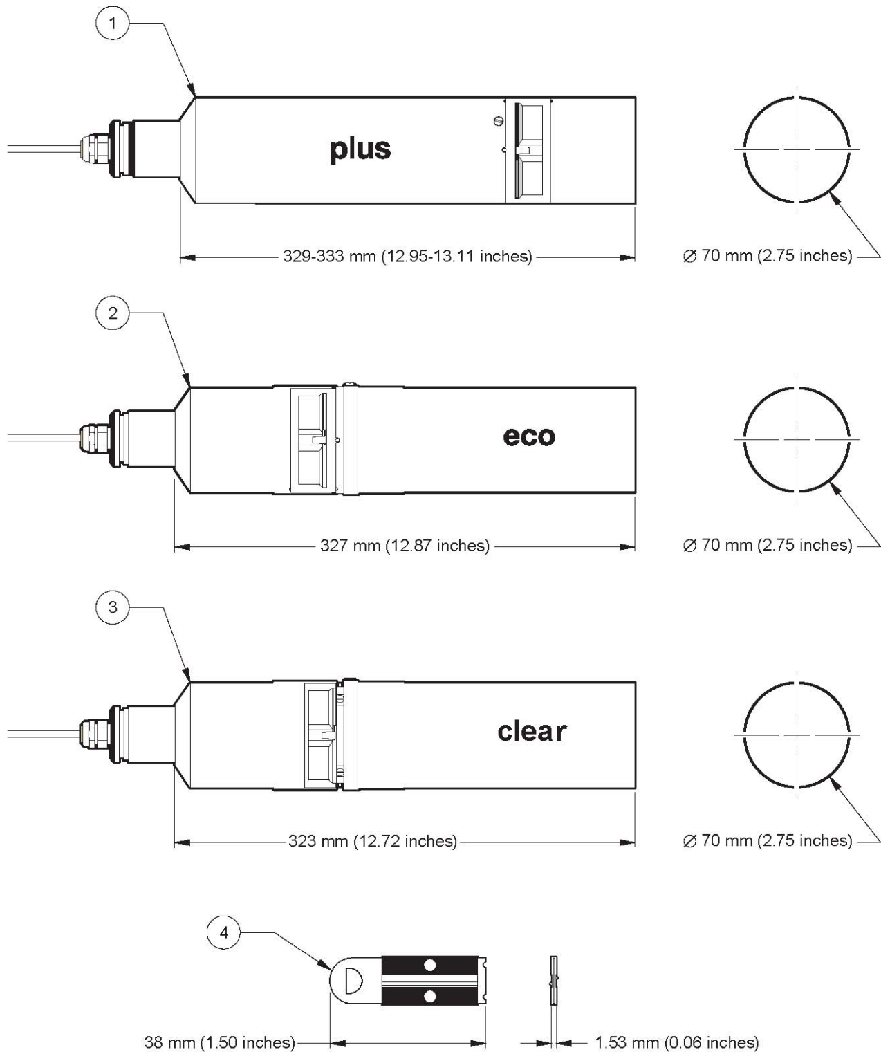
图24 传感器尺寸
