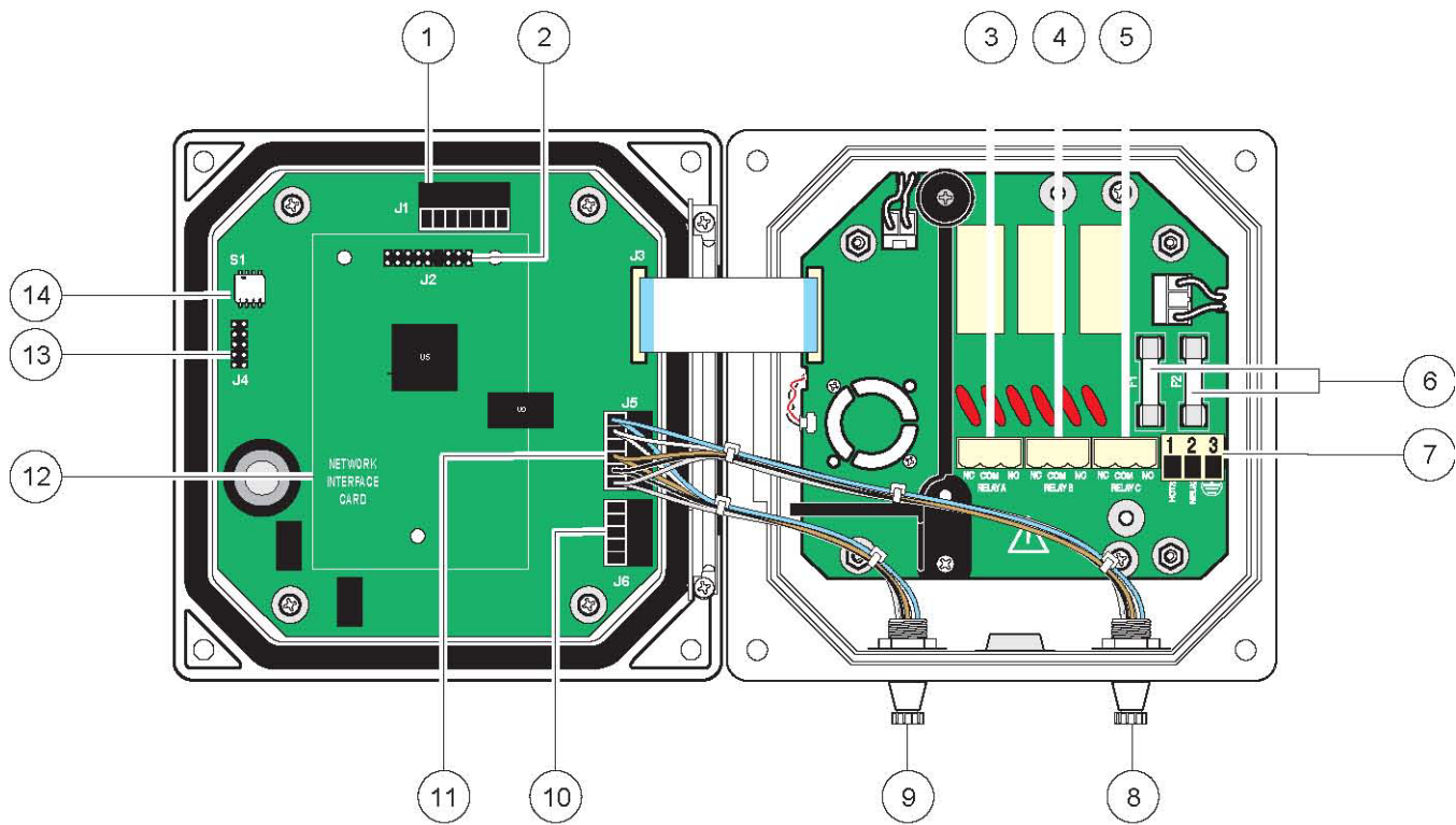
图15 导线连接
