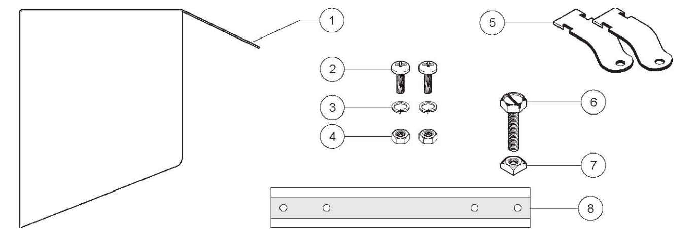
图7 遮阳罩的组成部件
