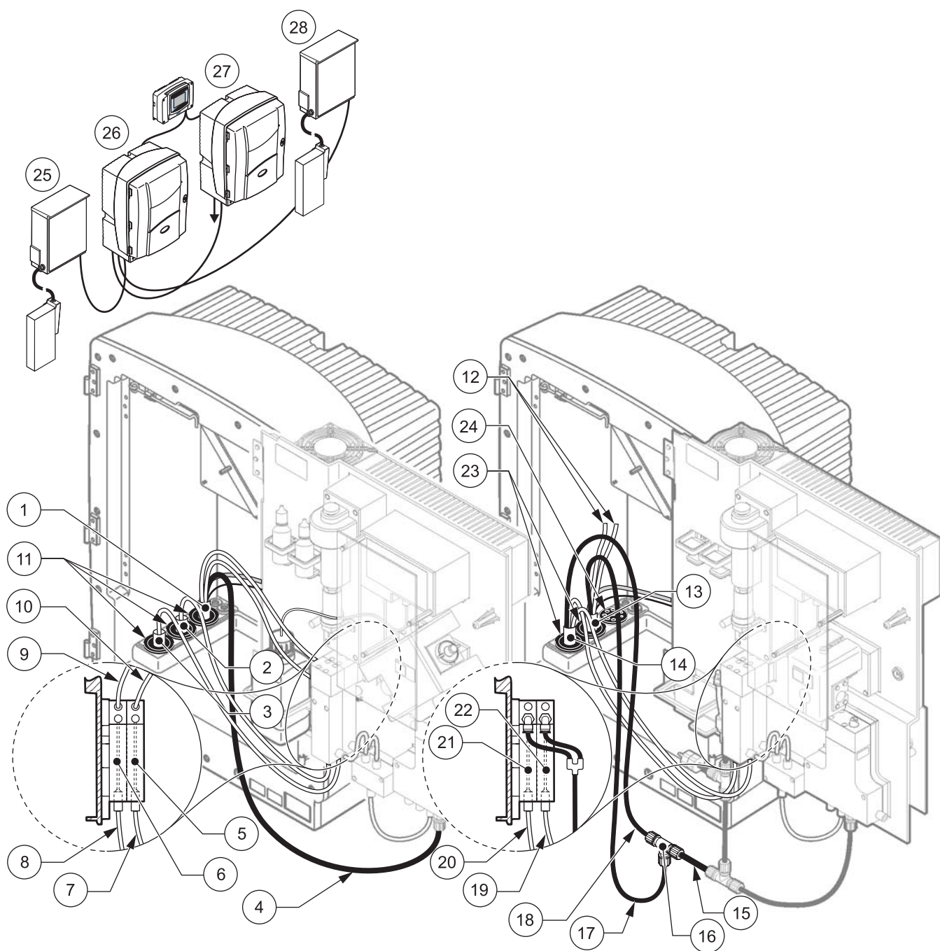
图 28 选项 6 设置
