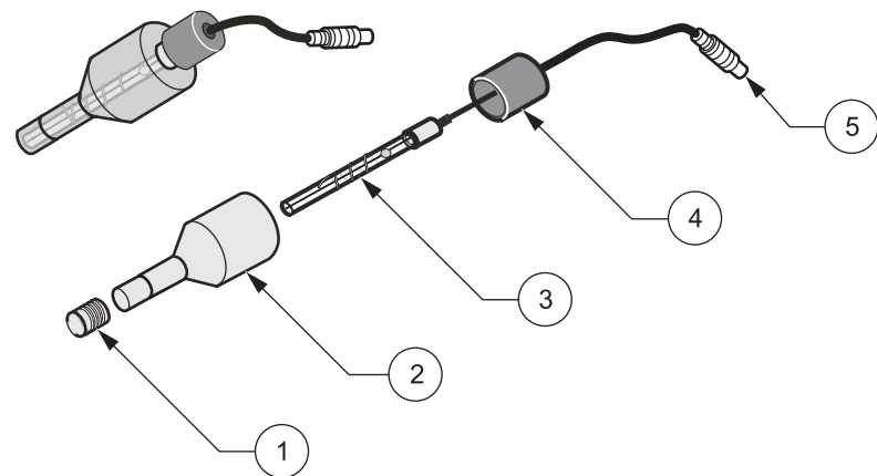
图 15 电极组件
