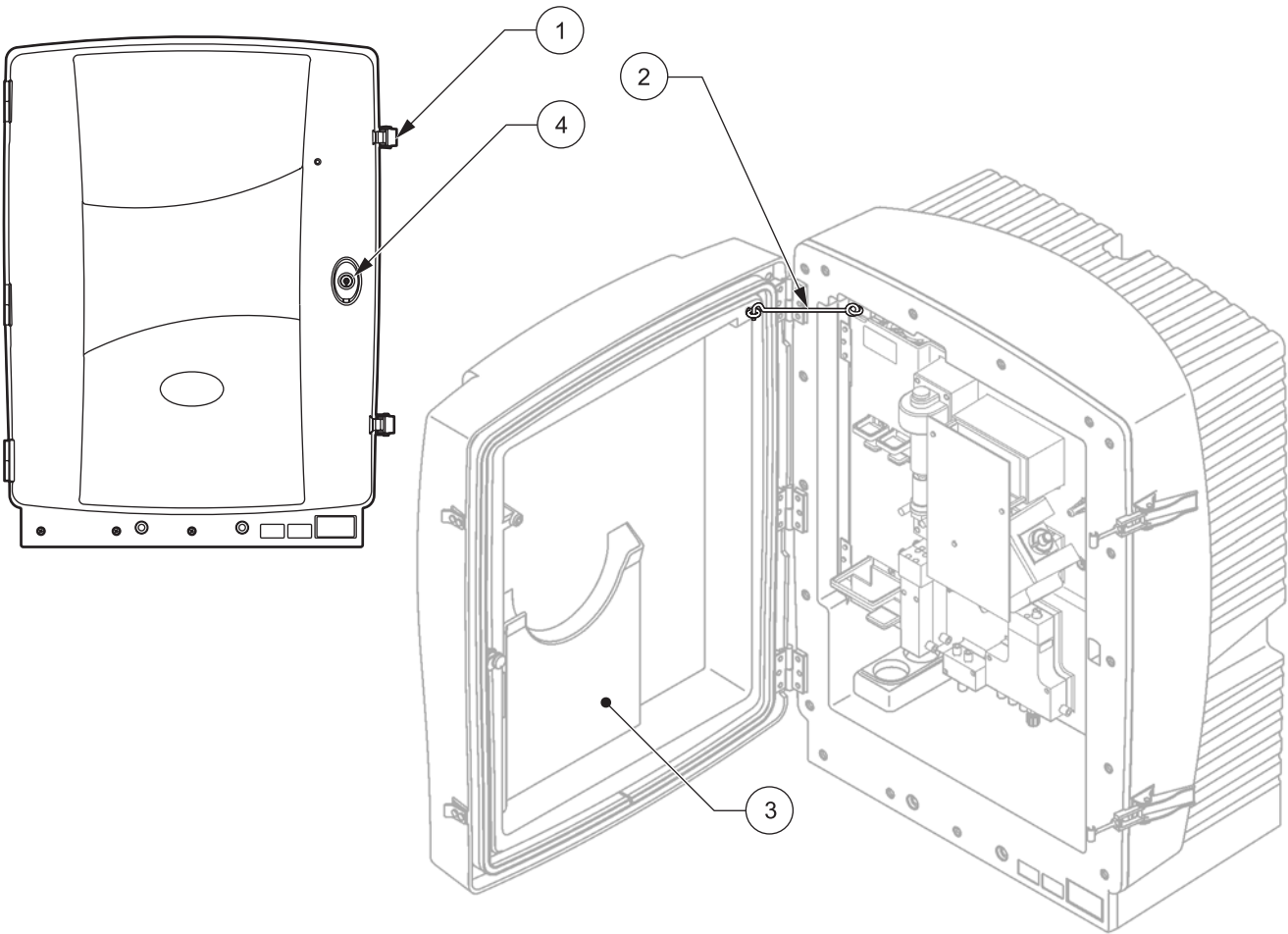
图 5 打开外壳
