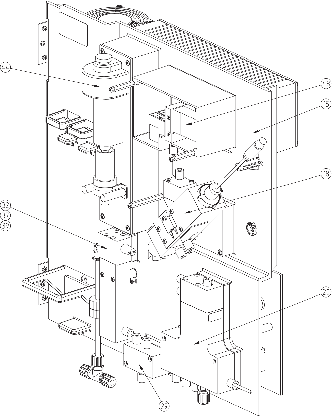
图 18 分析器面板概览
