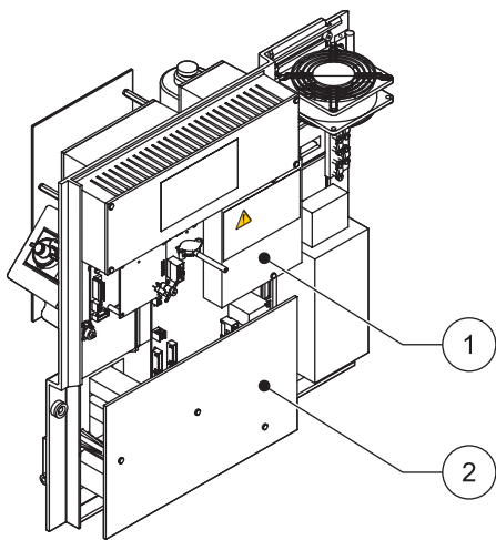
图 11 拆下防护罩
