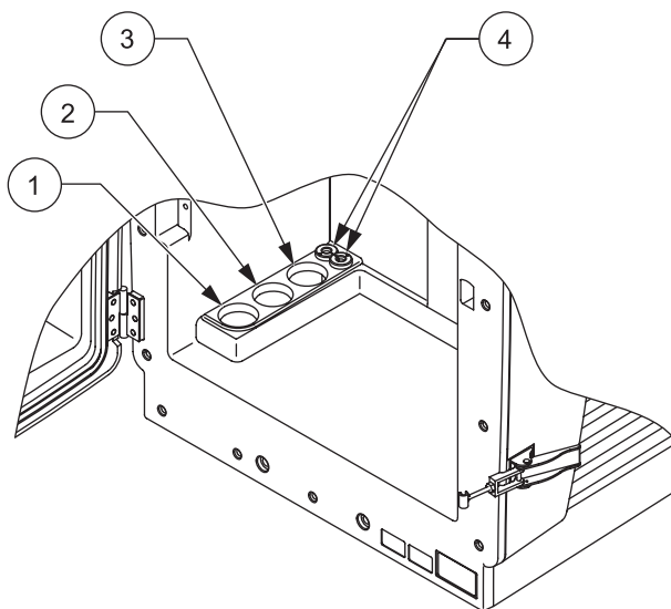
图 12 外壳开口
