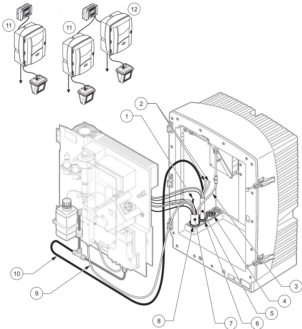
图 24 选项 2 设置
