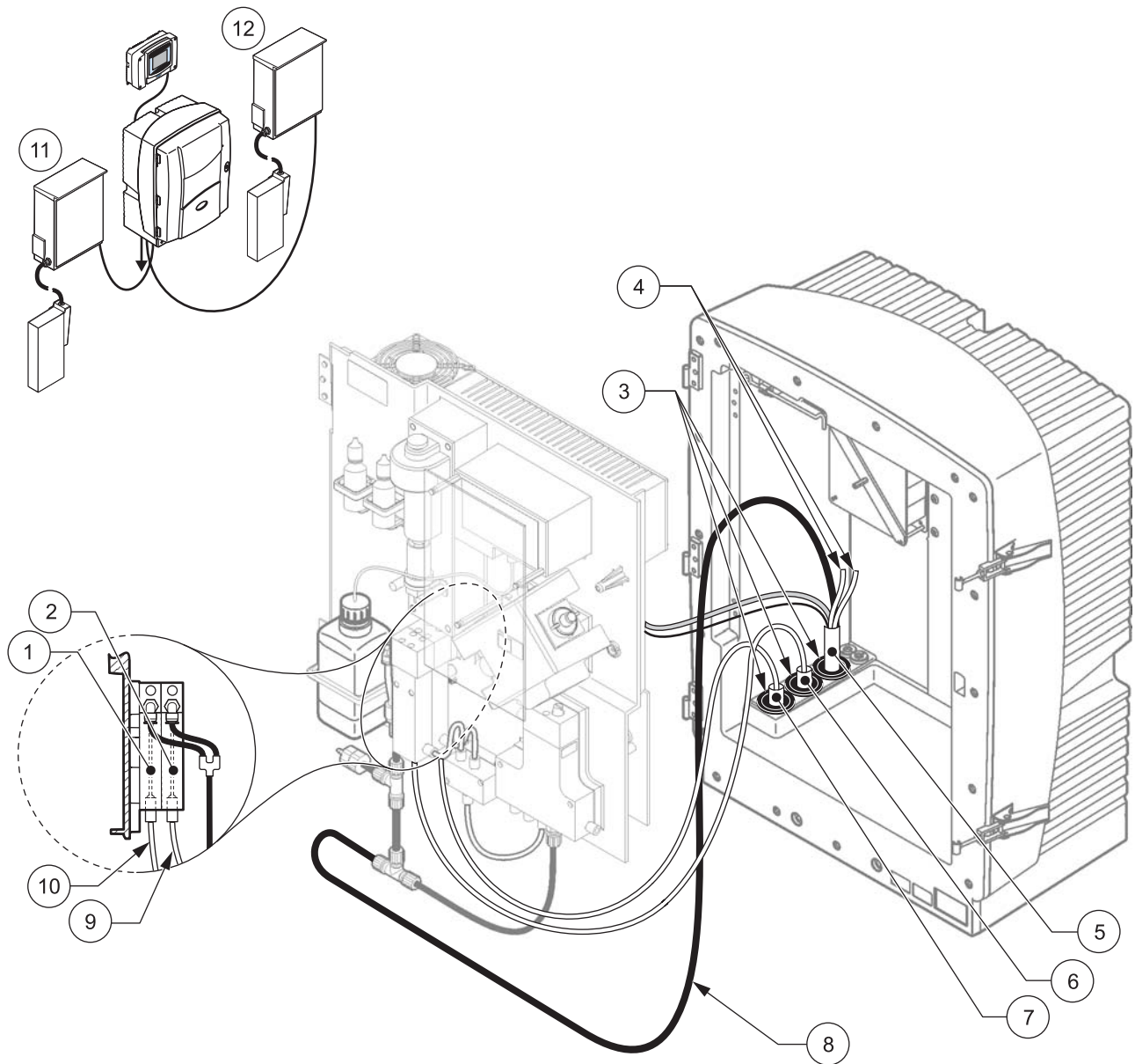
图 27 选项 5 设置
