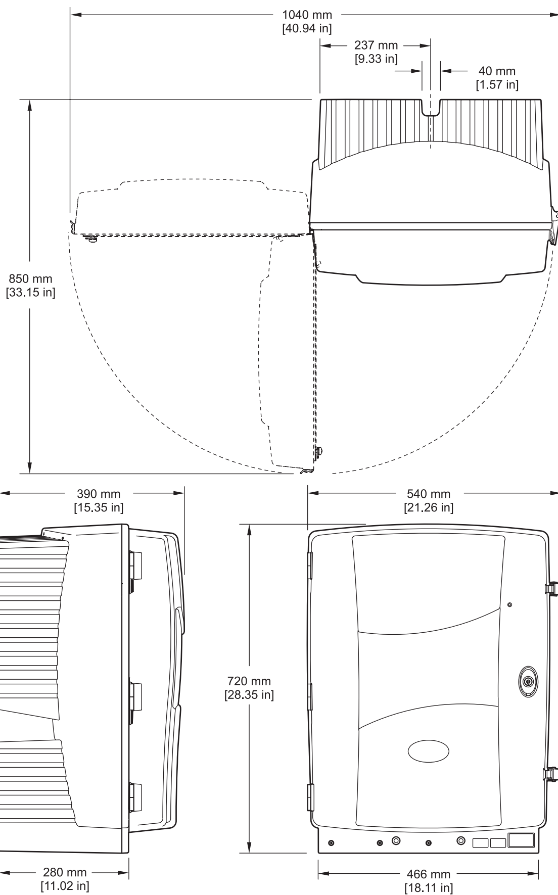
图 2 仪器尺寸
