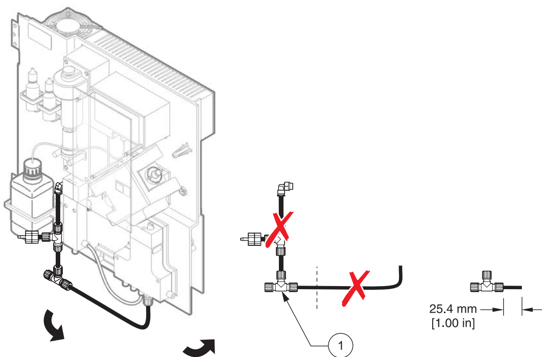
图 22 拆下 T 型连接装置
