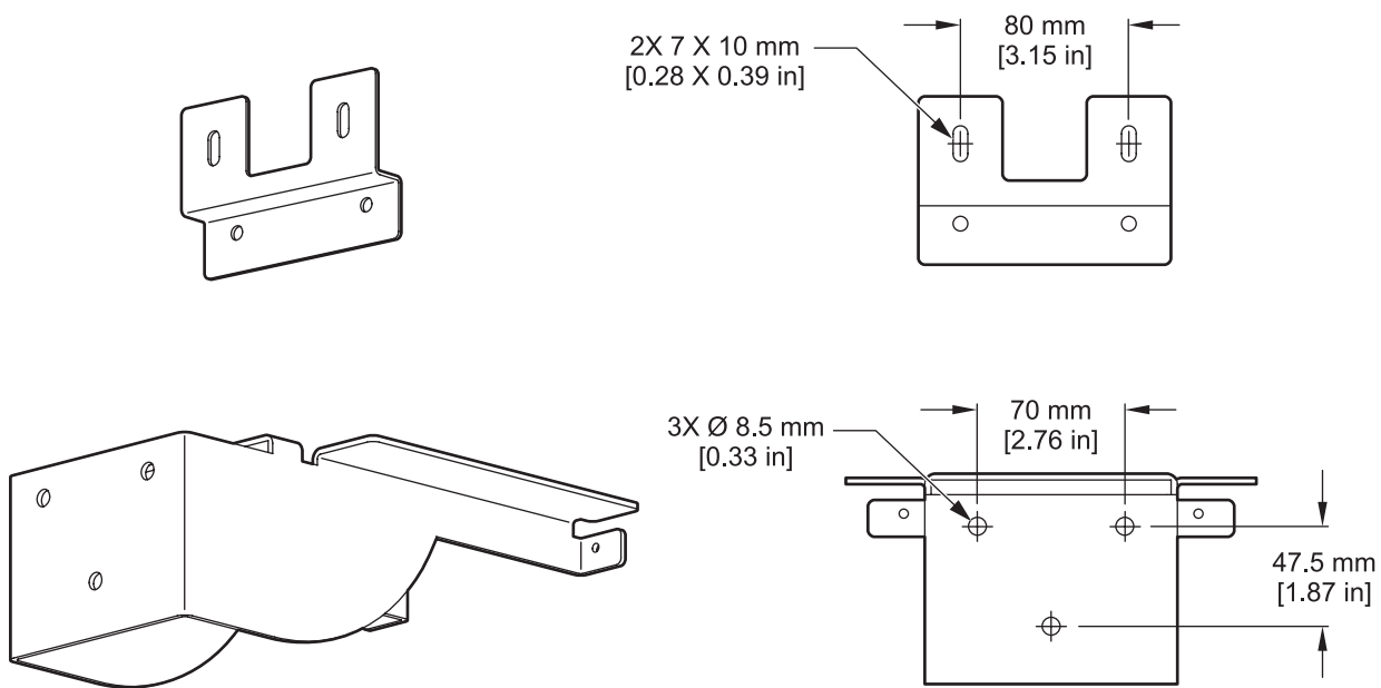
图 3 墙面安装的支架尺寸
